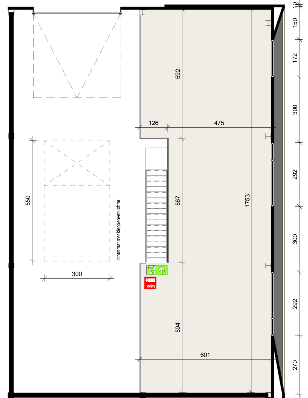
Verdieping 1
