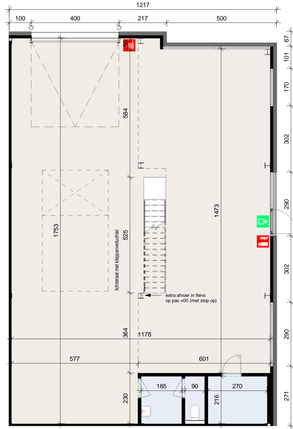
Gelijkvloers
