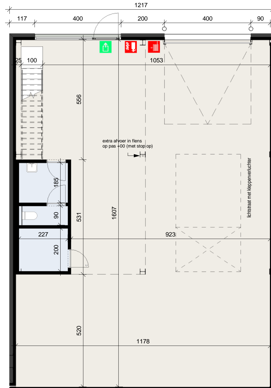
Gelijkvloers
