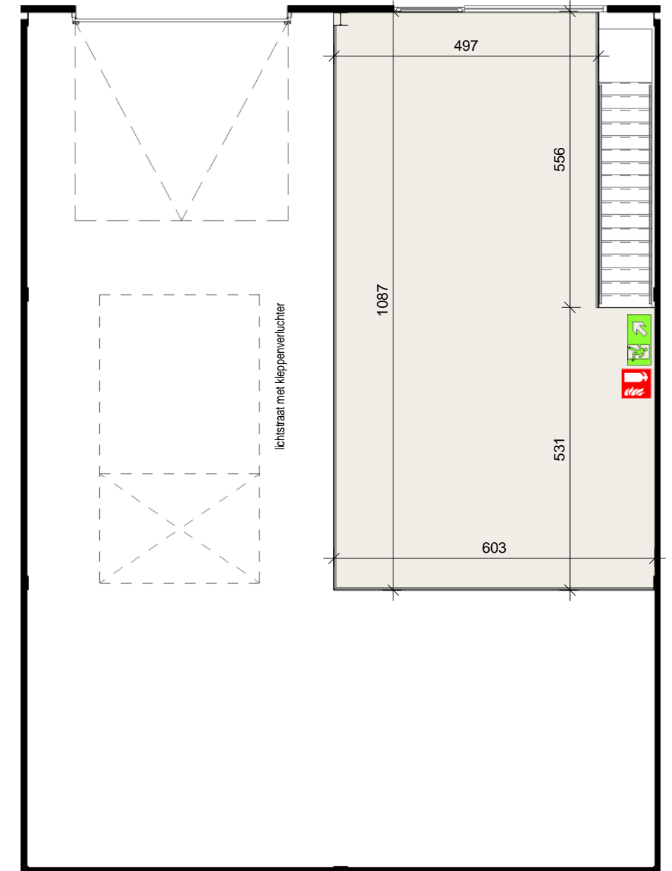
Verdieping 1
