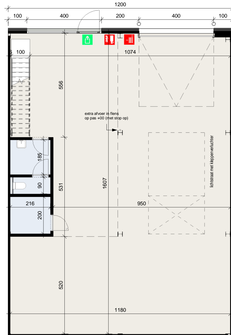
Gelijkvloers
