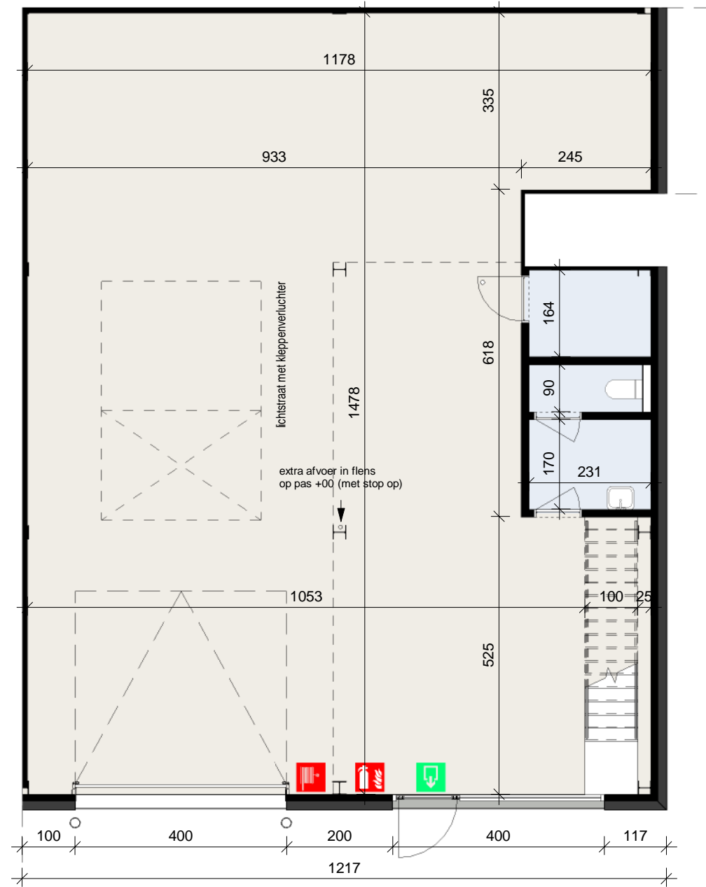
Gelijkvloers 1 : 100
