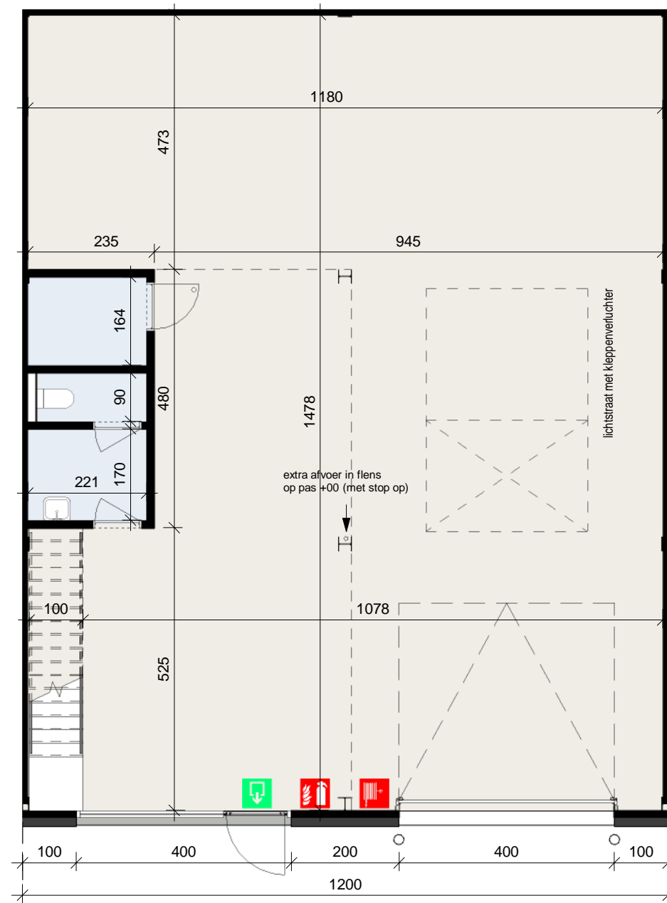
Gelijkvloers 1 : 100
