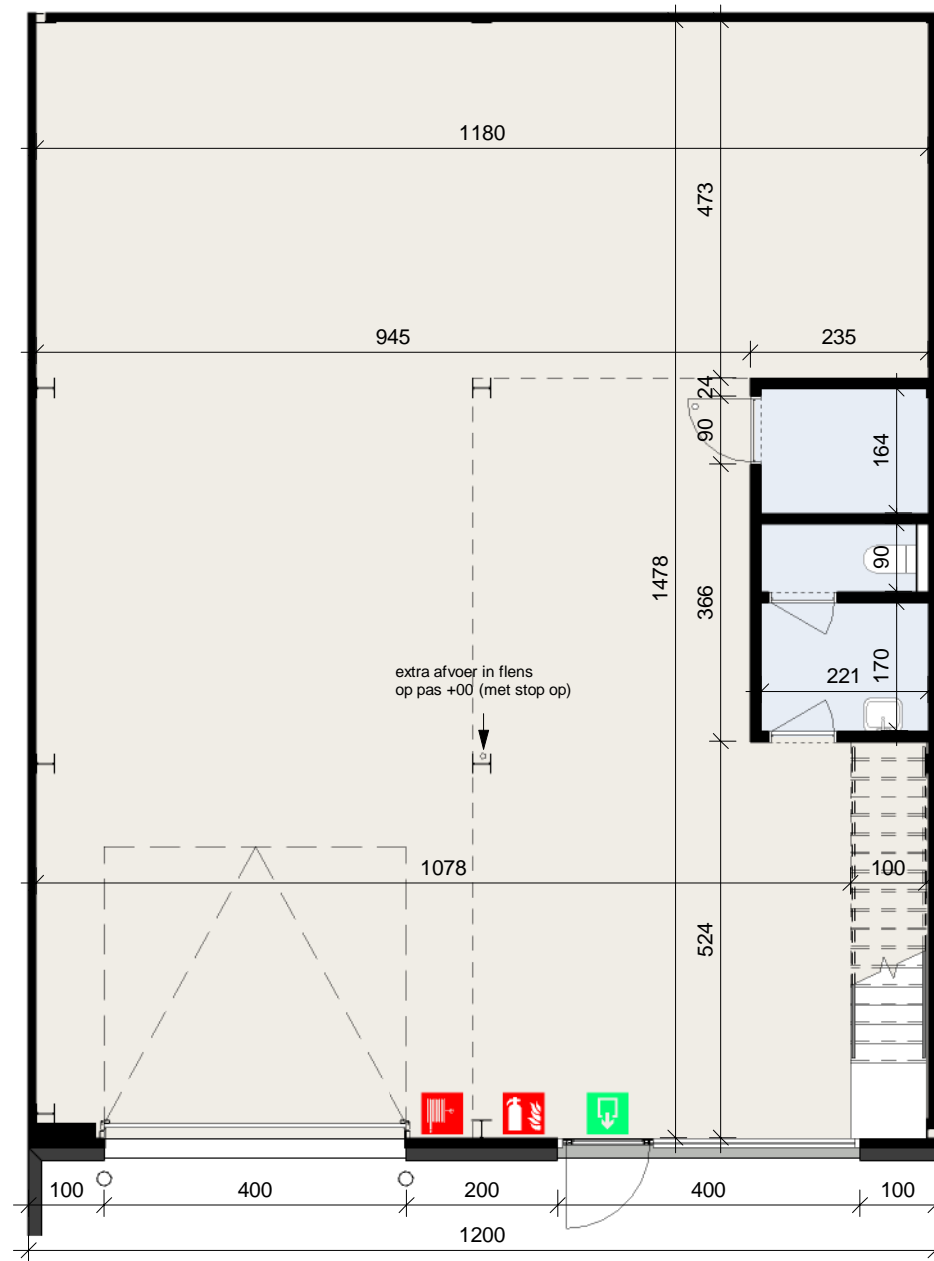
Gelijkvloers 1 : 100
