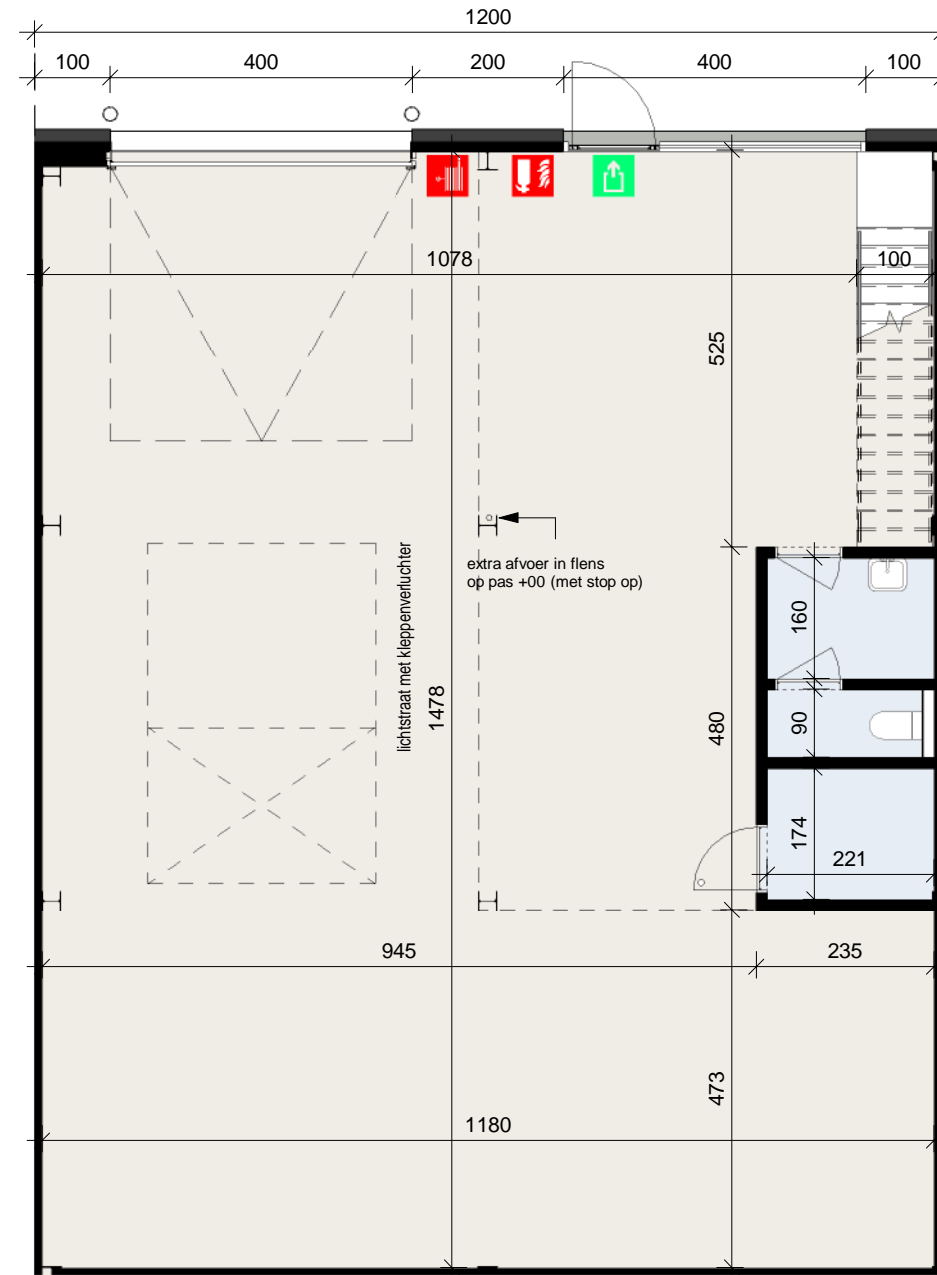
Gelijkvloers
