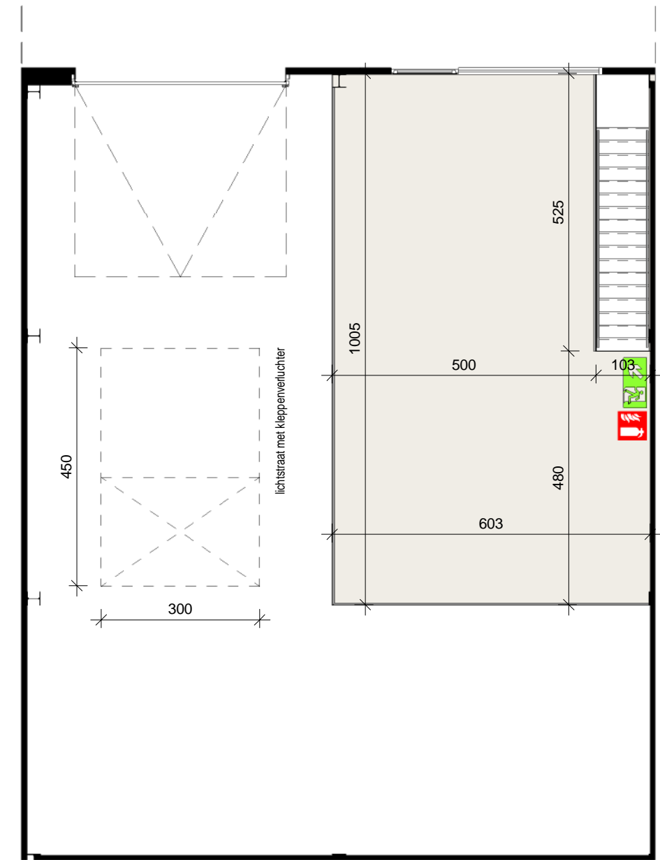
Verdieping 1
